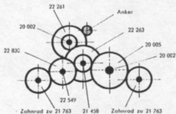
Fig. 4 Anordnung der Getrieberäder
