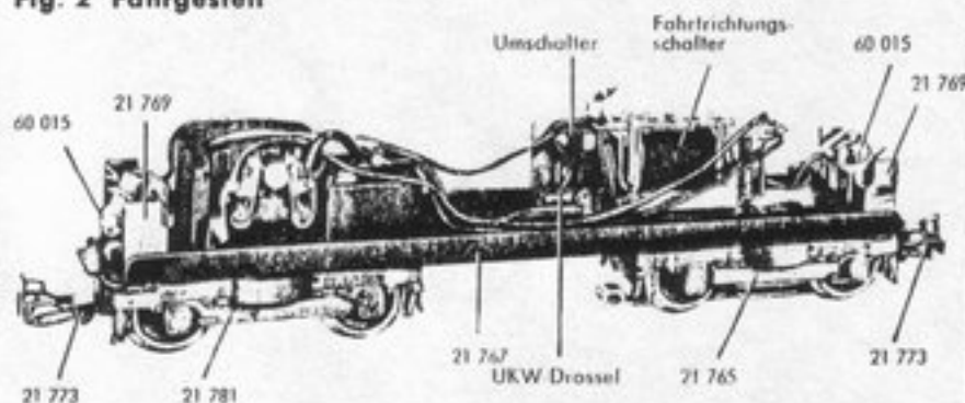
Fig. 2 Fahrgestell
