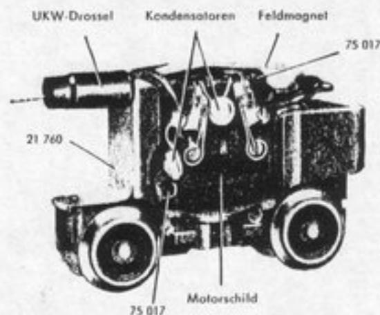
Fig. 3 Motordrehgestell
