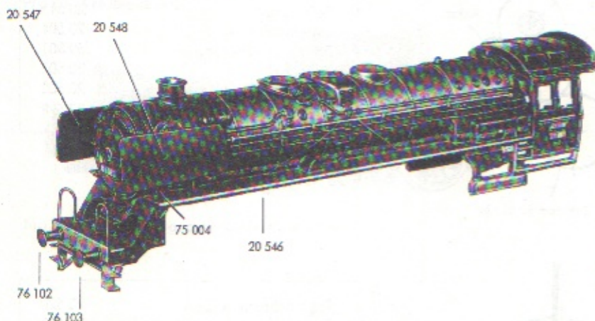
Fig. 1a Lampenhalter
