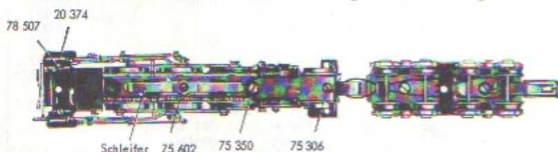
Fig. 2a Fahrgestelle (Lokomotive ohne Drehgestell, von unten gesehen)
