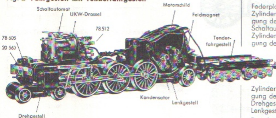
Fig. 2 Fahrgestell mit Tenderfahrgestell
