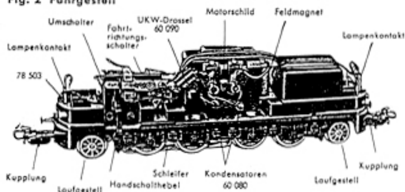
Fig. 2 Fahrgestell
