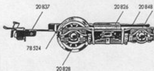
Fig. 6 Laufgestell
