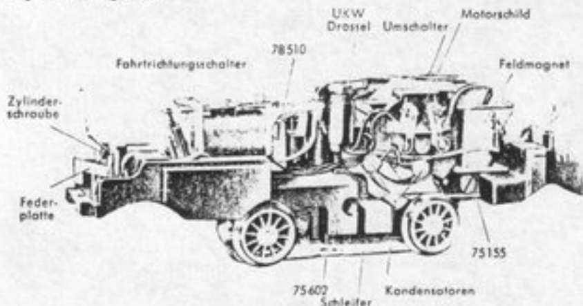
Fig. 3 Treibgestell
