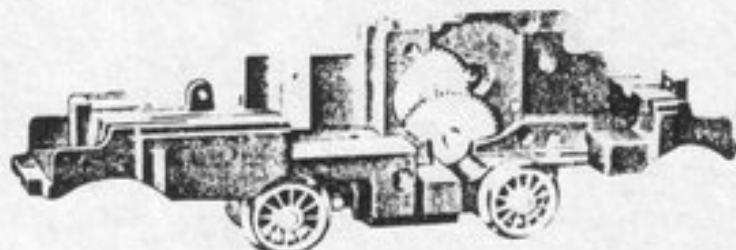
Fig. 3 Treibgestell
