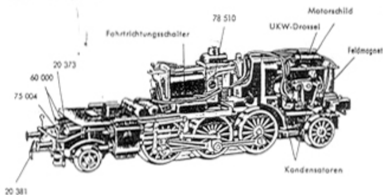
Fig. 2 Fahrgestell
