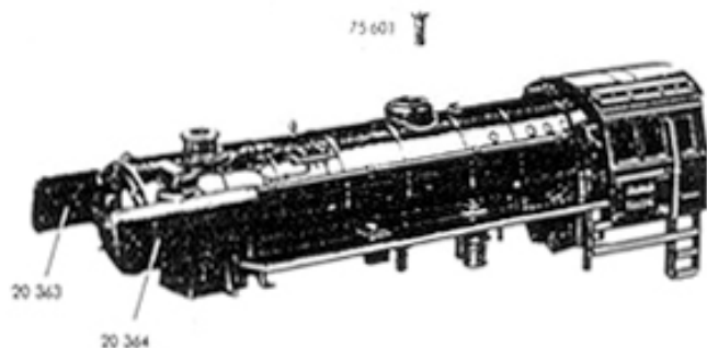
Fig. 1 Lokomotiv-Aufbau
