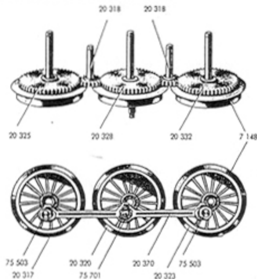
Fig. 5. Treibachsenteile und Treibräder
