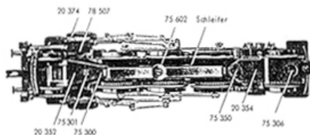
j. 2a Fahrgestell (von unten gesehen)
