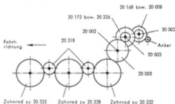
Fig. 4 Anordnung der Getrieberäder
