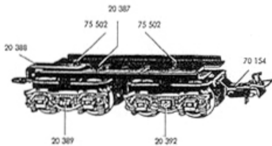
Fig. 2 Fahrgestell
